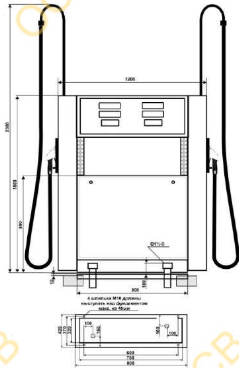
МОНТАЖНАЯ СХЕМА КОЛОНК "ШЕЛЬФ 100" 2 КЕД-50(90)-0,25-1-2
