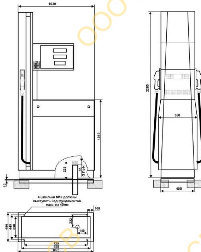
МОНТАЖНАЯ СХЕМА КОЛОНК "ШЕЛЬФ 200" 2 КЕД-50(90)-0,25-1-1
