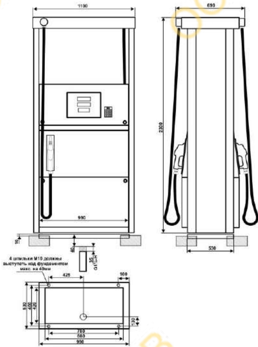
МОНТАЖНАЯ СХЕМА КОЛОНОК "ШЕЛЬФ 300" 2 КЕД-50(90)-0,25-2-1
