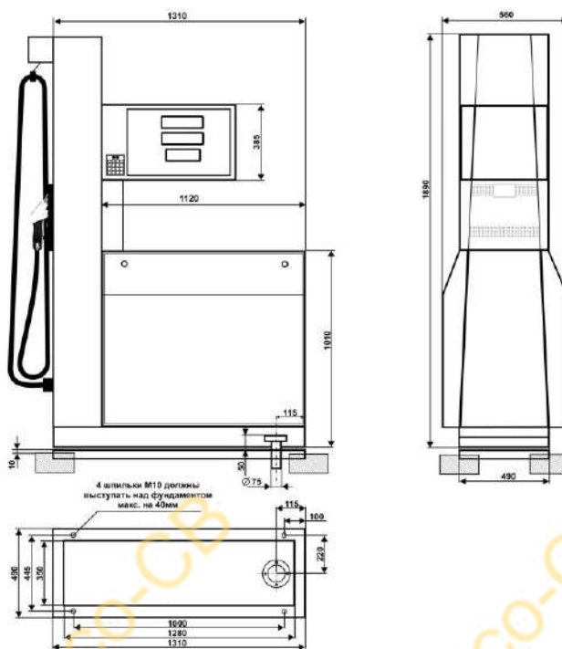
МОНТАЖНАЯ СХЕМА КОЛОНОК "ШЕЛЬФ 100" 1 КЕД-300-0,25-2-1
