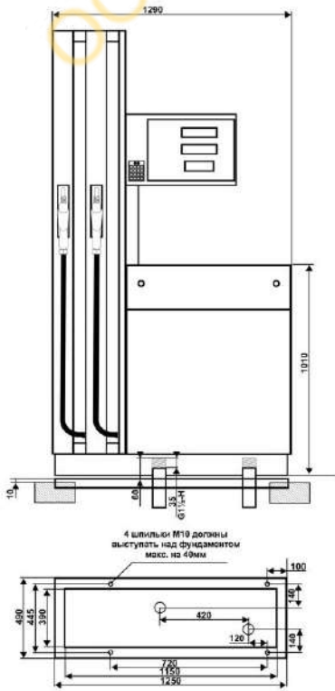
МОНТАЖНАЯ СХЕМА КОЛОНОК “ШЕЛЬФ 200” 2 КЕД-50(90)-0,25-2-2
