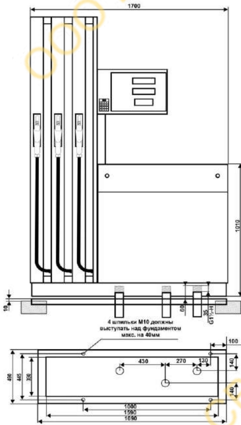
МОНТАЖНАЯ СХЕМА КОЛОНОК “ШЕЛЬФ 200” 2 КЕД-50(90)-0,25-2-3
