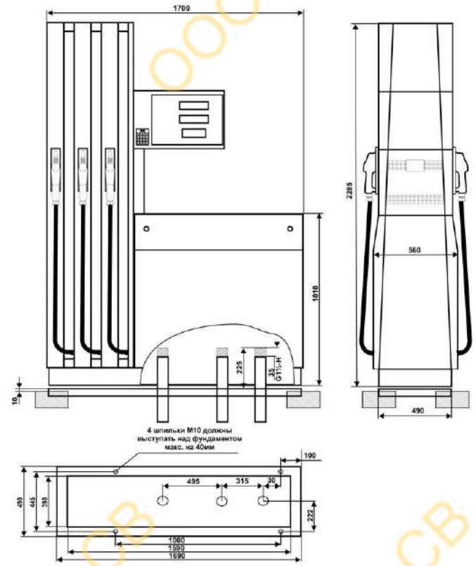
МОНТАЖНАЯ СХЕМА КОЛОНОК “ШЕЛЬФ 200” 2 КЕД-50(90)-0,25-1-3
