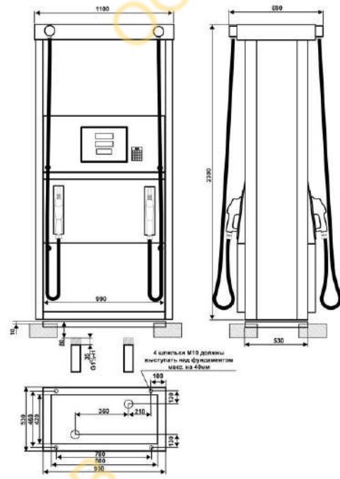
МОНТАЖНАЯ СХЕМА КОЛОНОК "ШЕЛЬФ 300" 2 КЕД-50(90)-0,25-2-2
