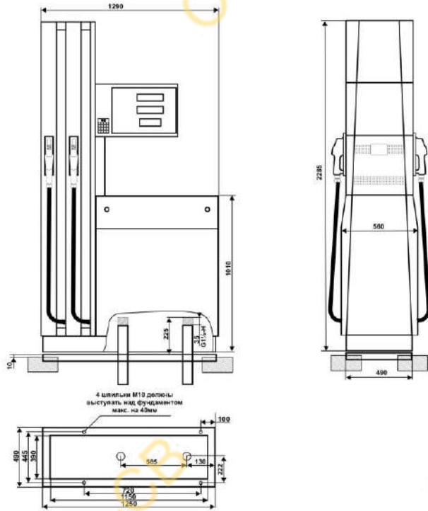
МОНТАЖНАЯ СХЕМА КОЛОНОК “ШЕЛЬФ 200” 2 КЕД-50(90)-0,25-1-2
